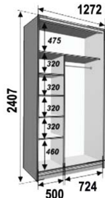
Двухдверный шкаф 1272
