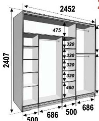
Четырехдверный шкаф 2452
