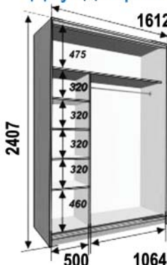
Двухдверный шкаф 2142
