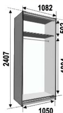
Двухдверный шкаф 1082
